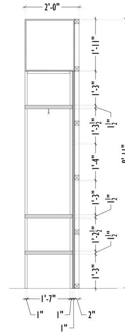
SECTION A-A'
